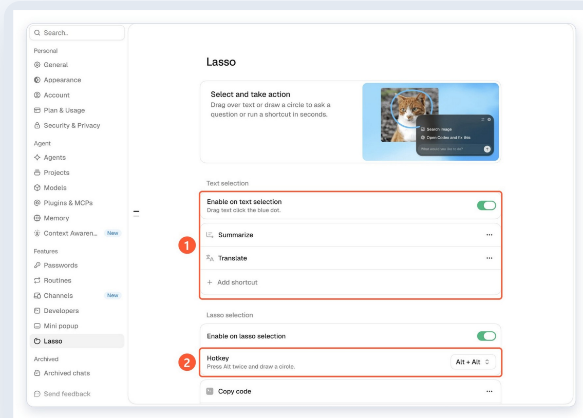
그림 5 · 설정 → Lasso → Add shortcut
